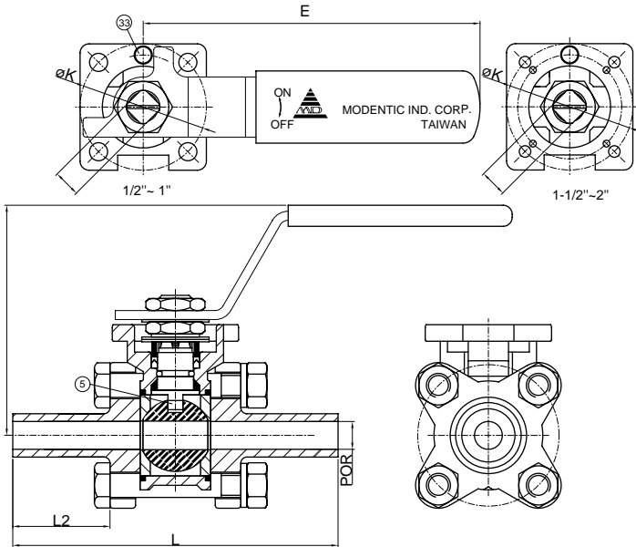
Fig No:MD-928EB US DIMENSIONS 1/2" - 4" DN15 ~ DN100
